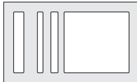
Linien 1
