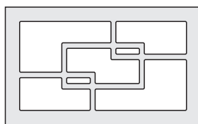
Linien 2
